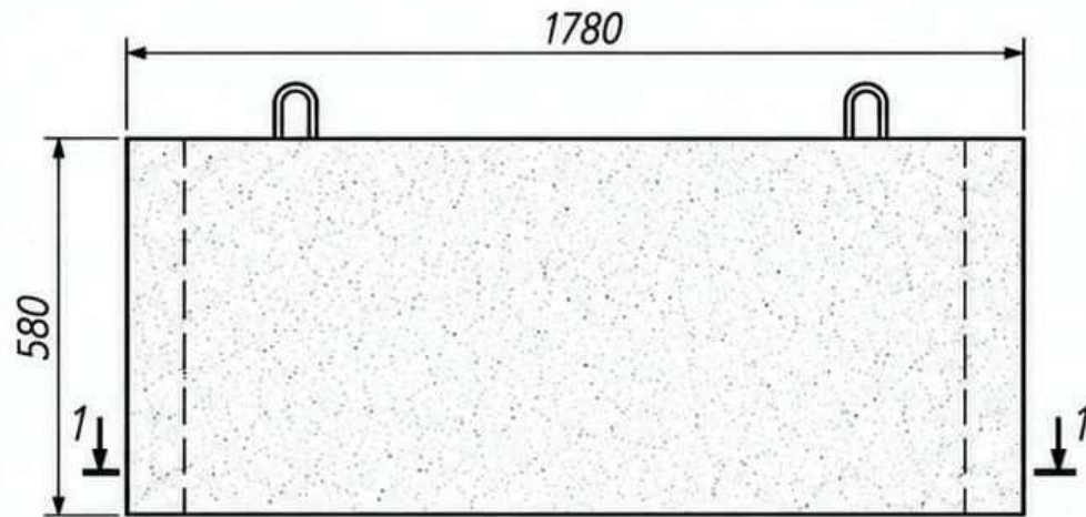
Вид спереди
