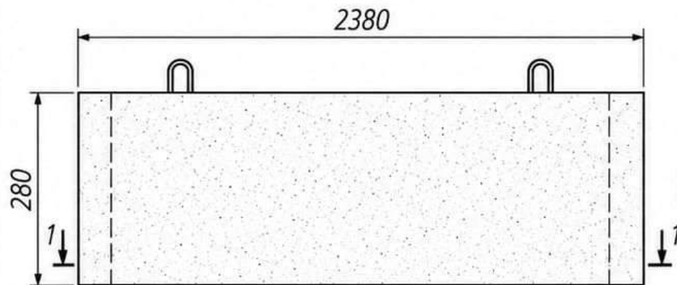
Вид спереди
