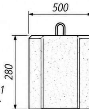
Вид сбоку
