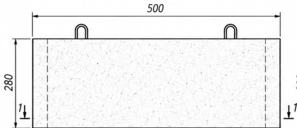
Вид спереди
