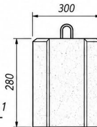
Вид сбоку
