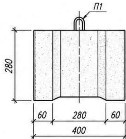
Вид сбоку
