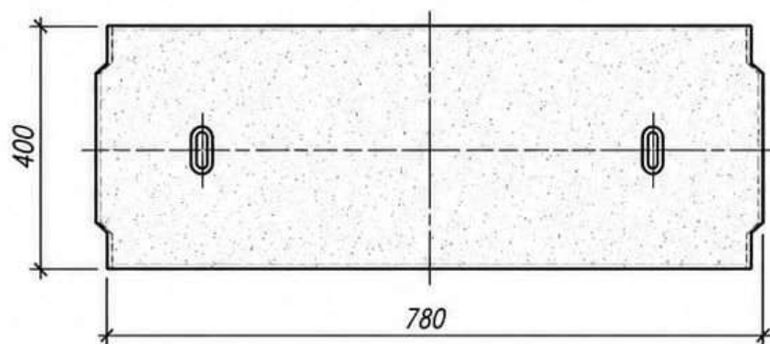
Вид сверху
