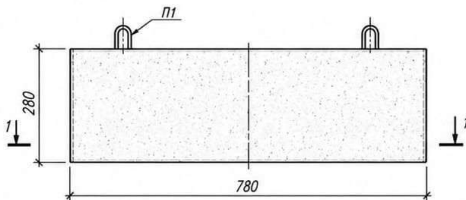
Вид спереди
