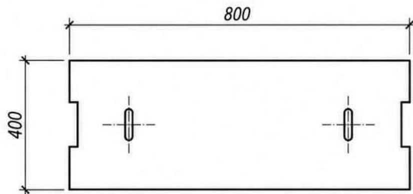
Вид сверху
