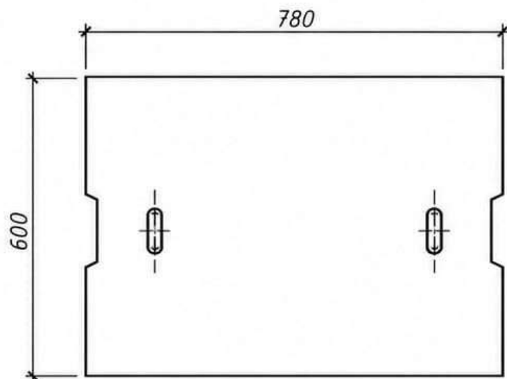
Вид сверху
