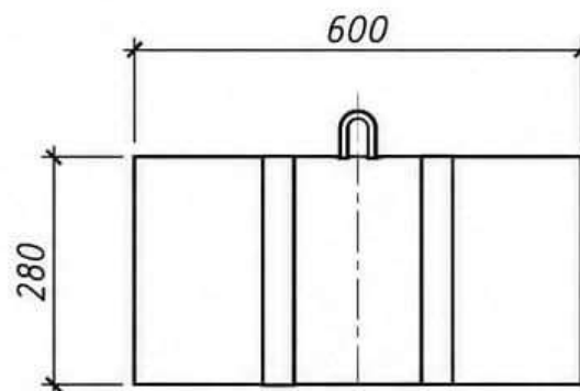
Вид сбоку
