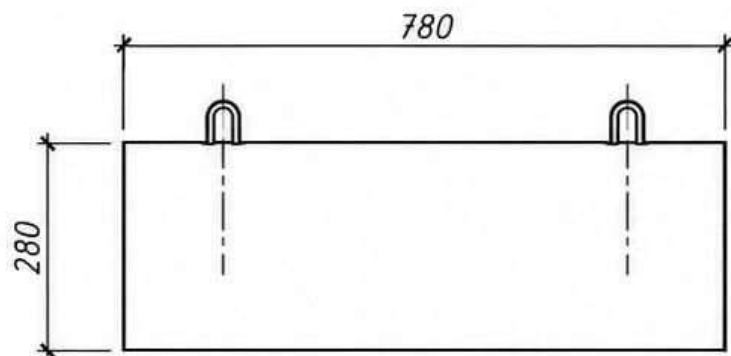
Вид спереди
