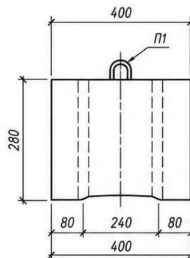
Вид сбоку
