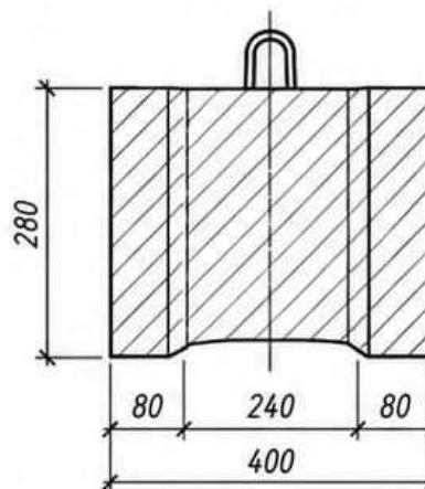
Разрез 1-1
