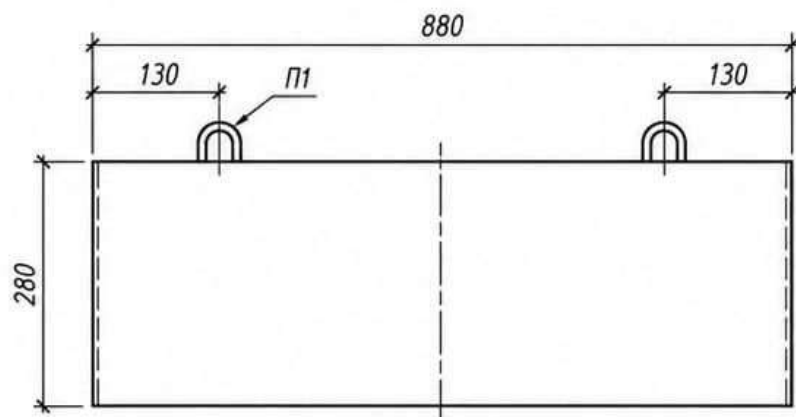
Вид спереди
