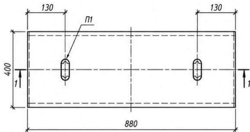
Вид сверху
