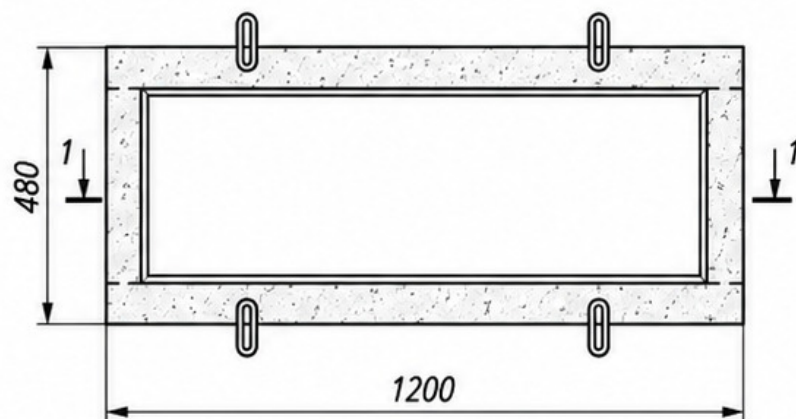
Вид сверху
