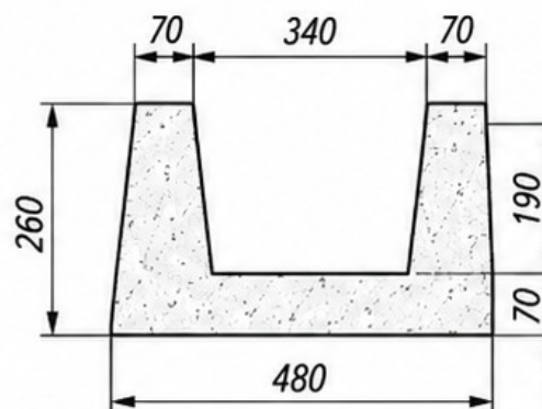
Сечение 1-1
