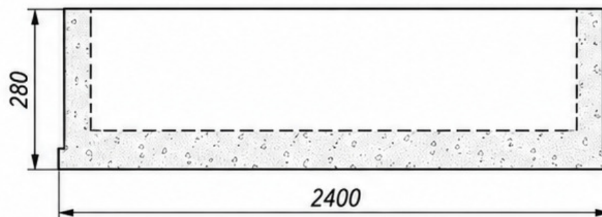
Вид сбоку
